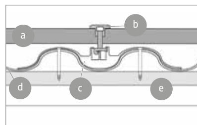
Horizontaler Schnitt, Quermontage
